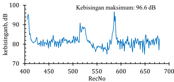
Gambar 5 Grafik kebisingan di titik 1
