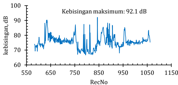
Gambar 7 Grafik kebisingan titik 3
