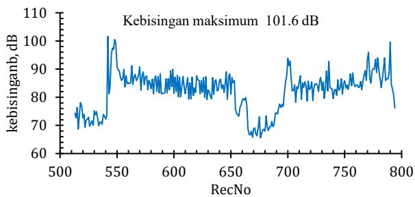
Gambar 6 Grafik kebisingan di titik 2.
