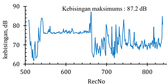
Gambar 8 Grafik kebisingan titik 4
